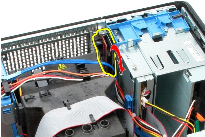
7. I/O パネルをスロットから持ち上げます。
